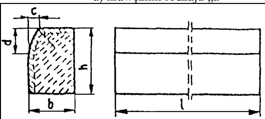
Rys. 1. Wymiarowanie krawężników
