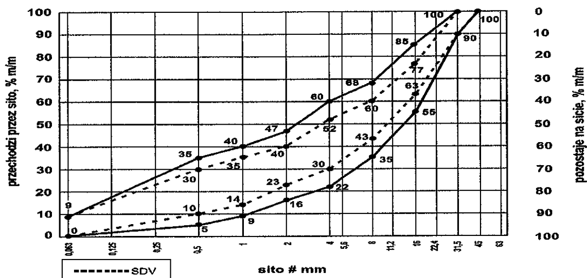
Rys. 1. Krzywe graniczne uziarnienia mieszanki kruszywo niezwiązanego 0/31,5 mm do warstw podbudowy zasadniczej
