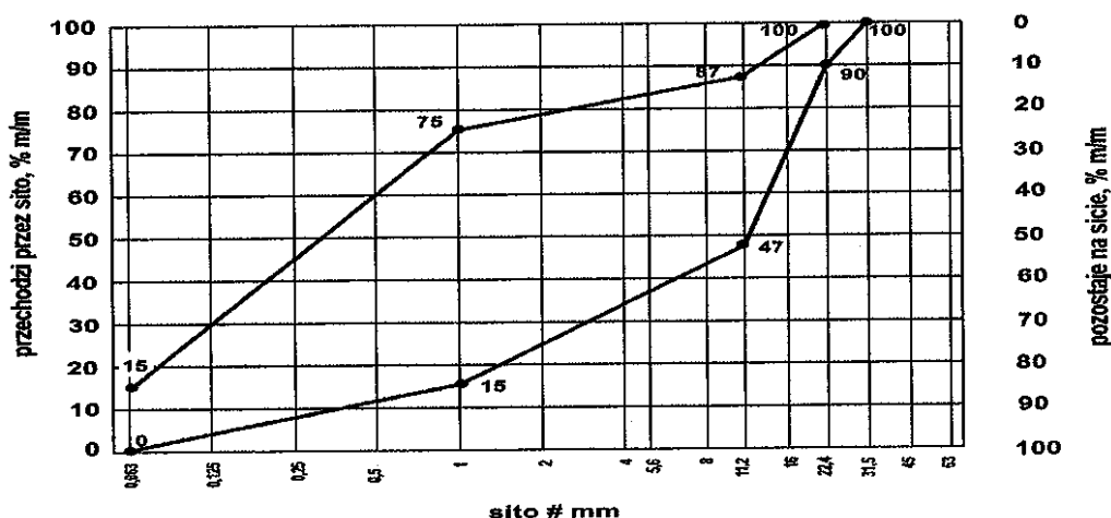
Rys. 1. Krzywe graniczne uziarnienia mieszanki kruszywa 0/22,4 mm do warstwy podłoża ulepszonego
