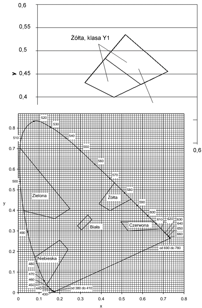
Rys.2. Współrzędne chromatyczności x,y dla barwy żółtej oznakowania
